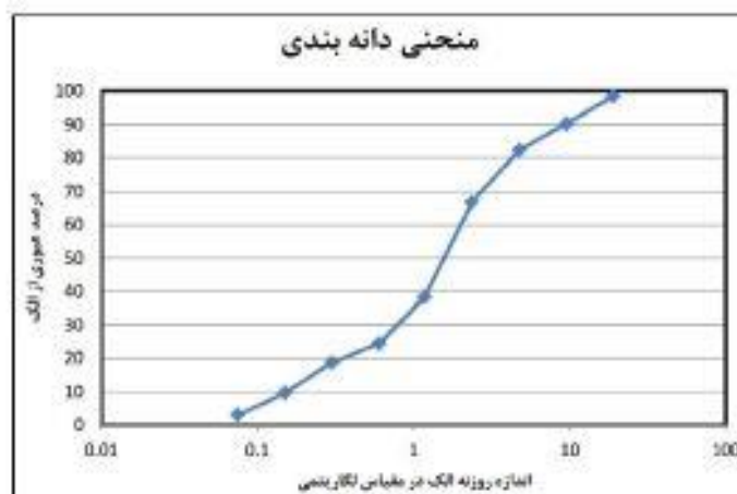
شکل ۱۶: منحنی دانه بندی
