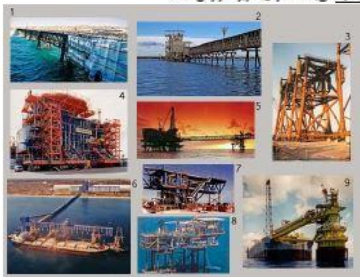
شکل ۹: سازه‌های دریایی
