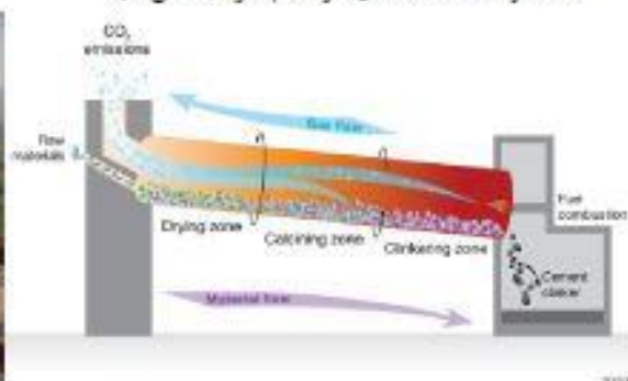
شکل ۴: کوره‌ی استوانه‌ای
