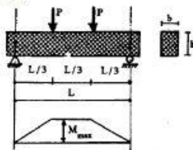
شکل ۲۰: آزمایش مقاومت خمشی بتن
