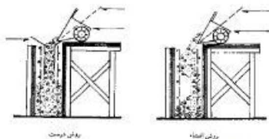
شکل ۳۴: بتن‌ریزی در ستون‌ها به وسیله‌ی قیف
