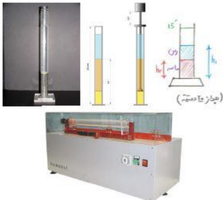
شکل ۱۱: آزمایش ارزش ماسه‌ای
