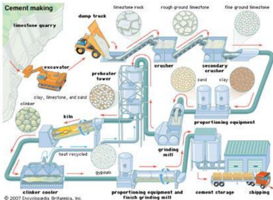
شکل ۶: مراحل تهیه سیمان در یک نگاه
