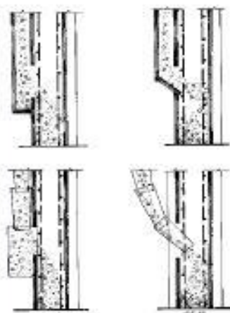
شکل ۳۳: بتن‌ریزی در ستون‌ها با تعبیه روزنه
