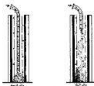
شکل ۳۲: بتن‌ریزی در ستون‌ها به وسیله‌ی پمپ بتن
