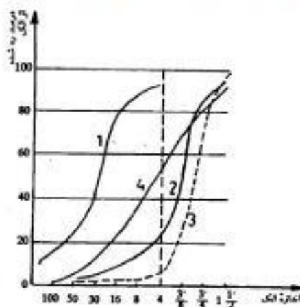
شکل ۱۵: نمونه‌هایی از منحنی دانه‌بندی
