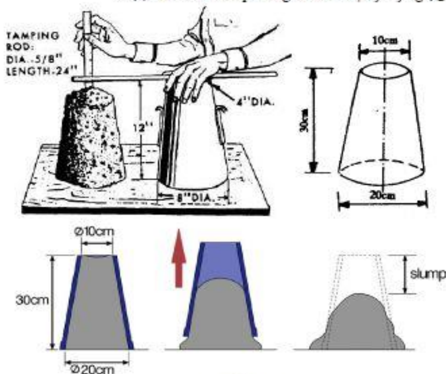
شکل ۲۰: آزمایش اسلامپ
