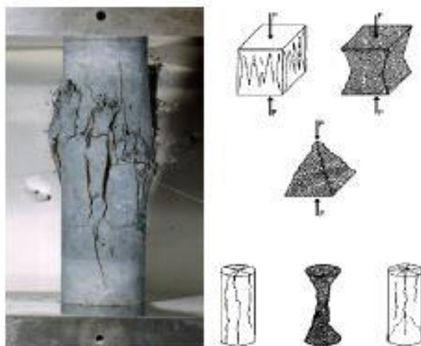
شکل ۲۶: آزمایش مقاومت فشاری بتن
