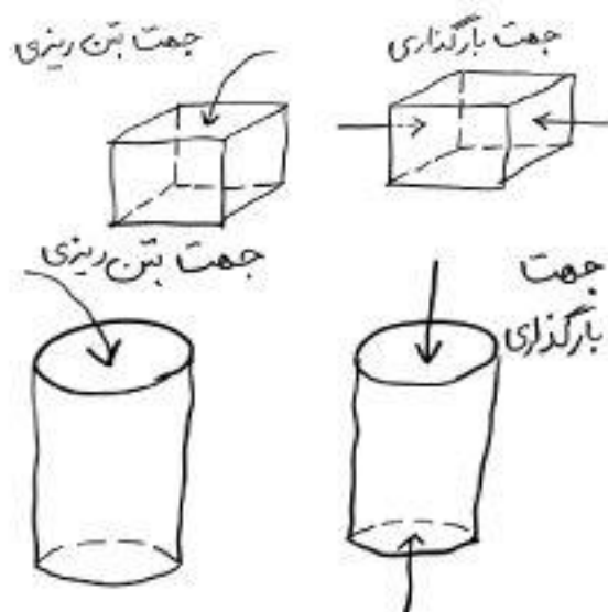
شکل ۲۷: جهت بارگذاری و بتن‌ریزی برای نمونه‌های استوانه‌ای و مکعبی
