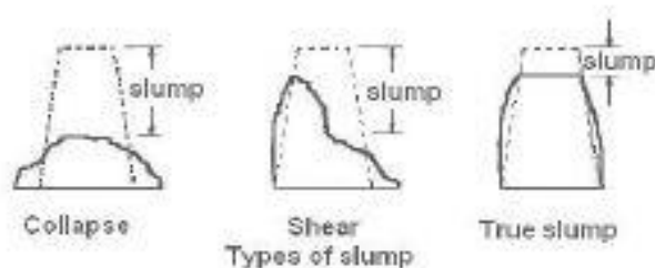
شکل ۲۱: حالات مختلف اسلامپ
